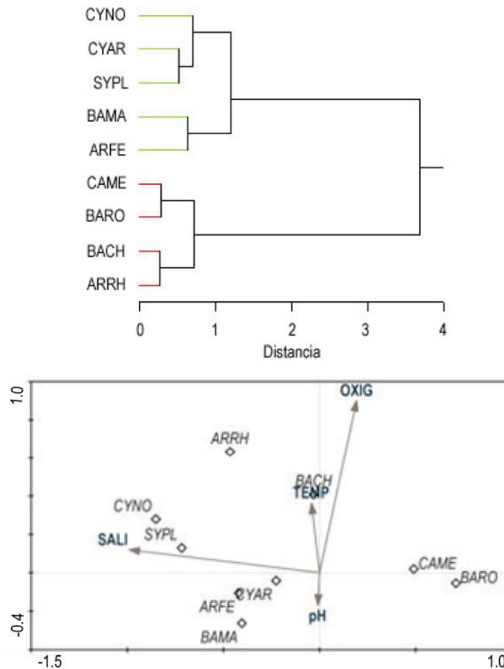
Figura 9. Cluster de asociación de especies dominantes (método Ward, distancia gamma) y análisis canónico de correspondencia de las especies dominantes con los parámetros ambientales. CYN0 ( Cynoscion nothus ), CYAR ( Cynoscion arenarius ), SYPL ( Symphurus plagiusa ), BAMA ( Bagre marinus ), ARFE ( Arius felis ), CAME ( Cathorops melanopus ), BARO ( Bairdiella ronchus ), BACH ( Bairdiella chrysoura ) ARR0 ( Archosargus rhomboidalis ), SALI (salinidad), TEMP (temperatura), OXIG (oxígeno disuelto).
